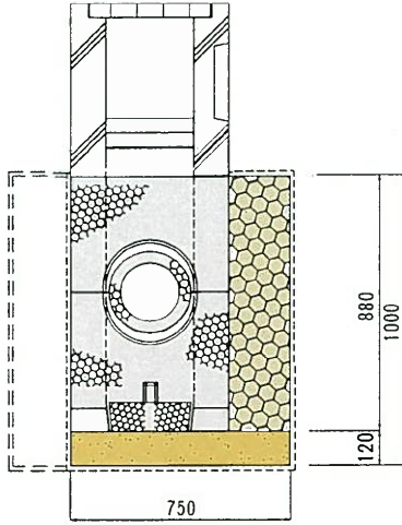
側面図
