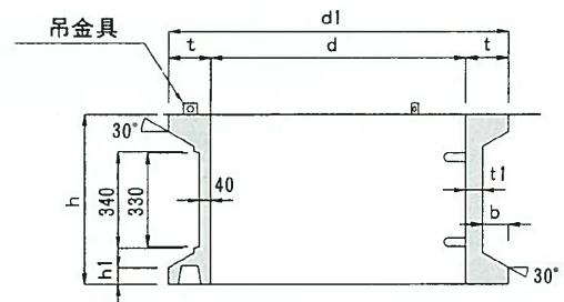
A-A 断面図
