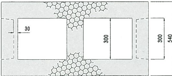
平面図
