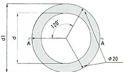
平面図
