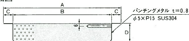
断面図
