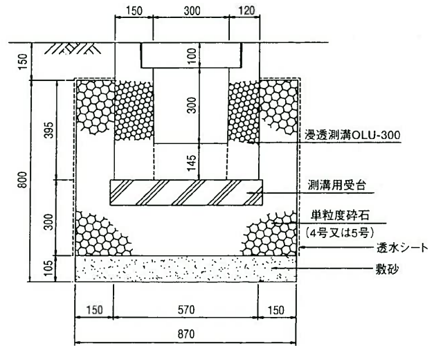
標準構造図
