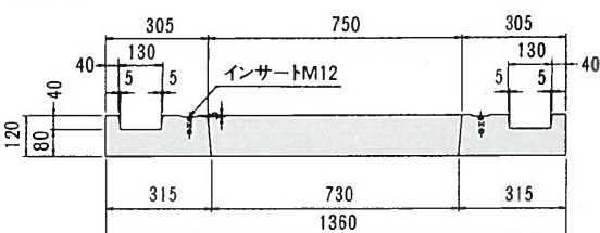
底板断面図
