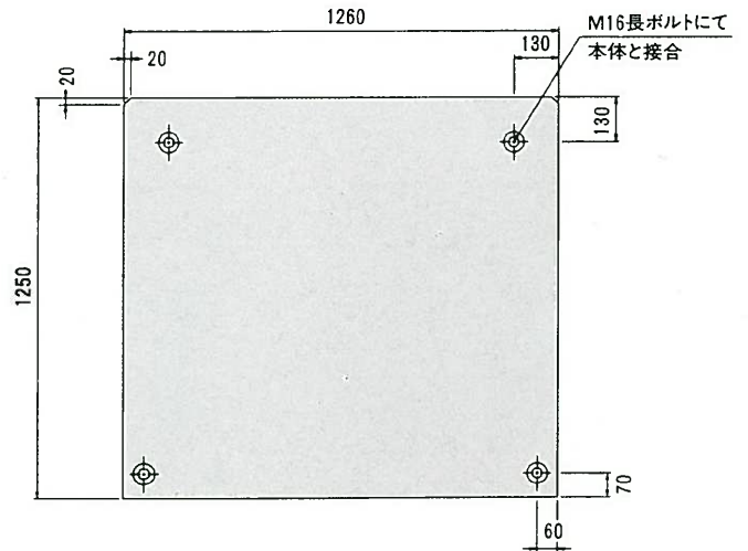
妻壁平面図
