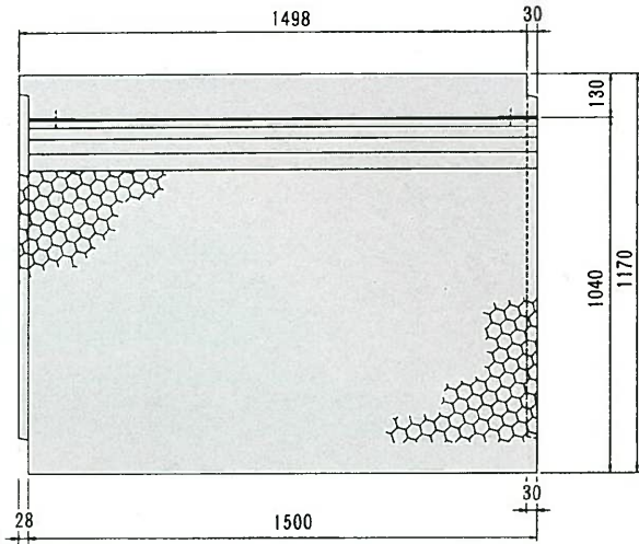
側面図
